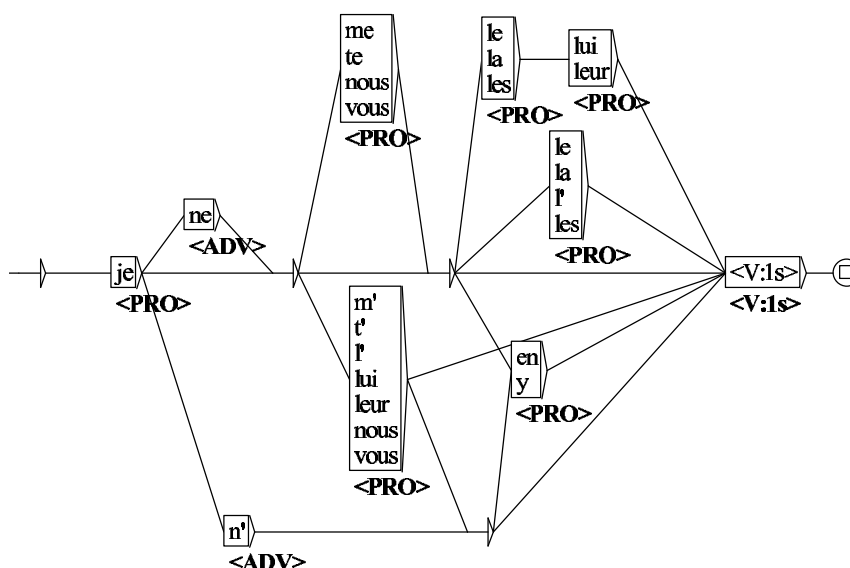
Figure 2 : Grammaire locale de désambigüisation : je plus verbe.grf.
